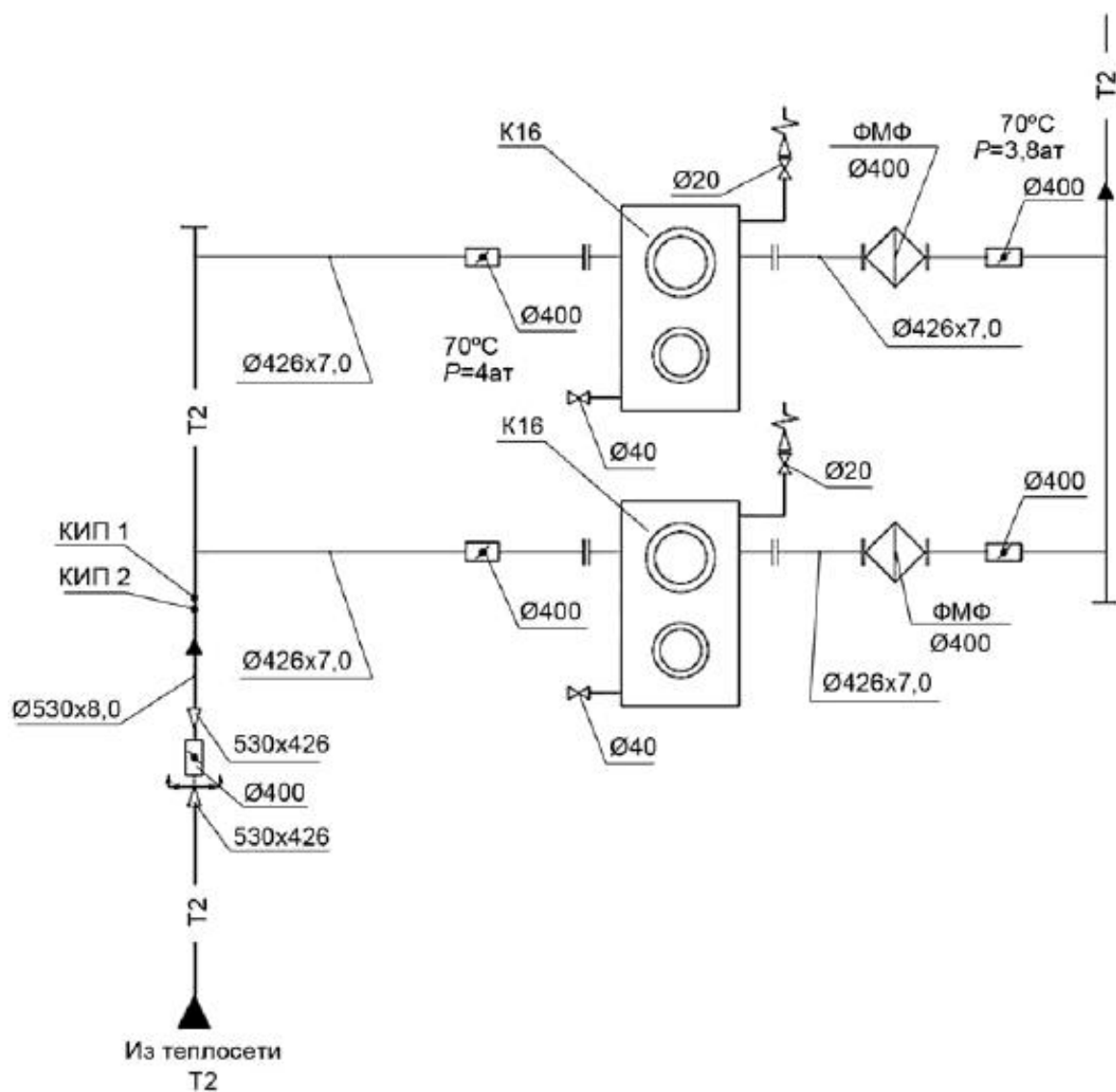
Рисунок Г.4 - Пример выполнения схемы установки грязевиков
