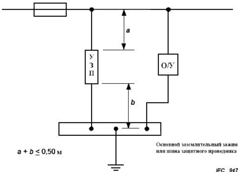
Рисунок 53D - Пример установки устройств защиты от перенапряжений на вводе электроустановки или рядом с ним
